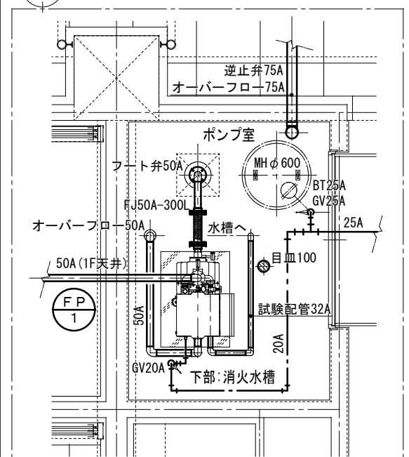
消火栓ポンプ室詳細図 1:50 消火水槽: 有効水量 2.6m³
